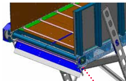
Självremsande drivhjul
