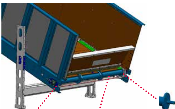
Självcentrerande lager
