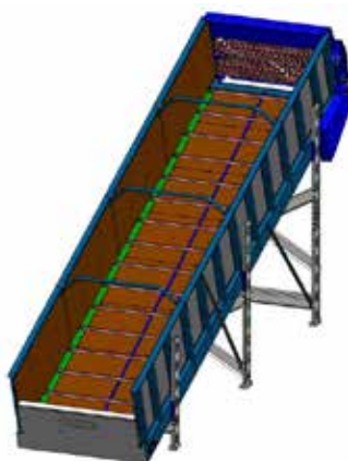
Silage Ripper
